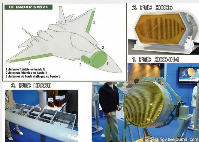
Архитектура многоэлементного бортового радиолокационного комплекса Н036 «Белка» (Ш-121) истребителя 5-го поколения Су-57.
