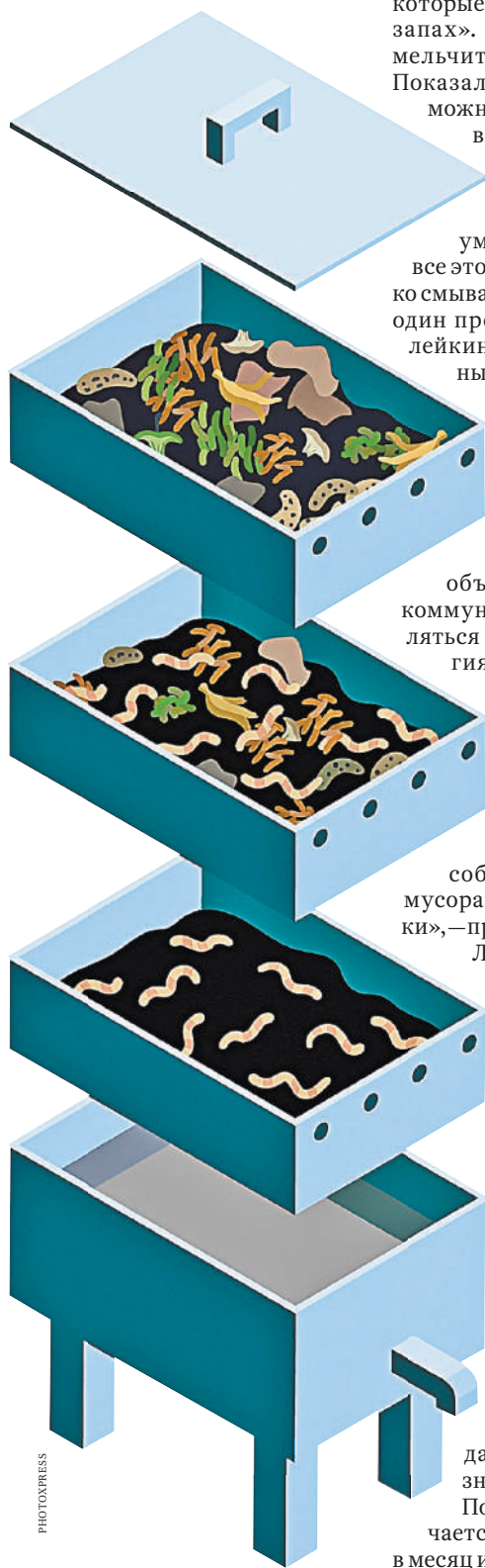
Вермиферма не занимает много места — контейнеры можно ставить один на другой.
