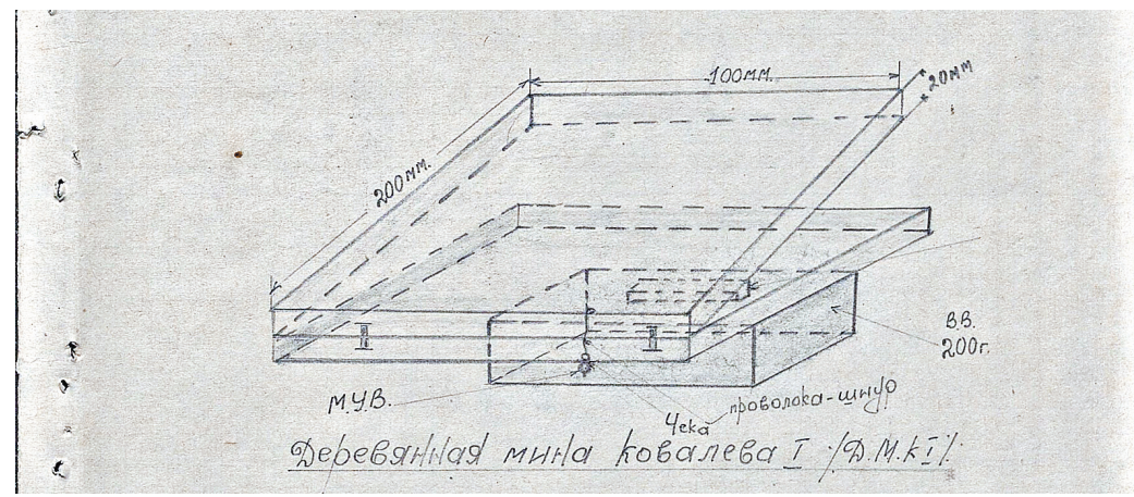
Схема «деревянной мины» Ковалева I (ДМ-К). М.У.В. — минный универсальный взрыватель мгновенного действия.
