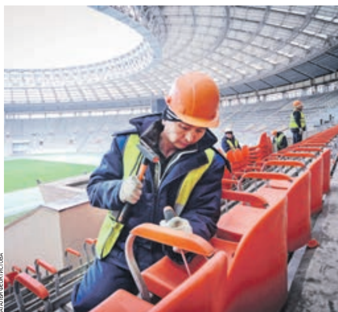
2014 год. Реконструкция Большой спортивной арены «Лужников» вступила в решающую стадию. Рабочие демонтируют старые кресла на трибунах для болельщиков
