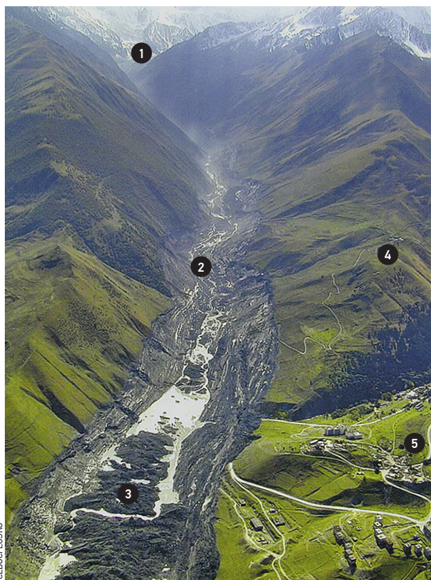
2002 год. Долина реки Геналдон после прохождения селя: 1 — ледник Майли, 2 — река Геналдон, 3 — тыловая часть завала, 4 — селение Тменика, 5 — поселок Кармадон
