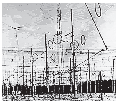
Многофункциональный радиокomплекс «Сура».
