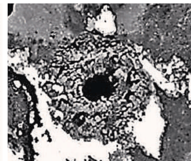
На фото слева, сделанном из космоса, — бугор пучения — наполненный метаном карман в слоях многовековой мерзлоты. На фото справа — воронка, образовавшаяся от его прорыва.
