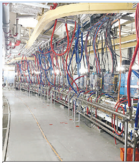
Система магнитов, установленная на накопительное кольцо СКИФа.
