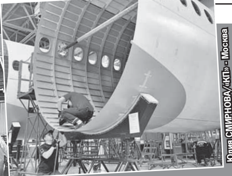
Будущие лайнеры МС-21-310. Их обещают сделать очень удобными для пассажиров - с просторным салоном и большими багажными полками.
