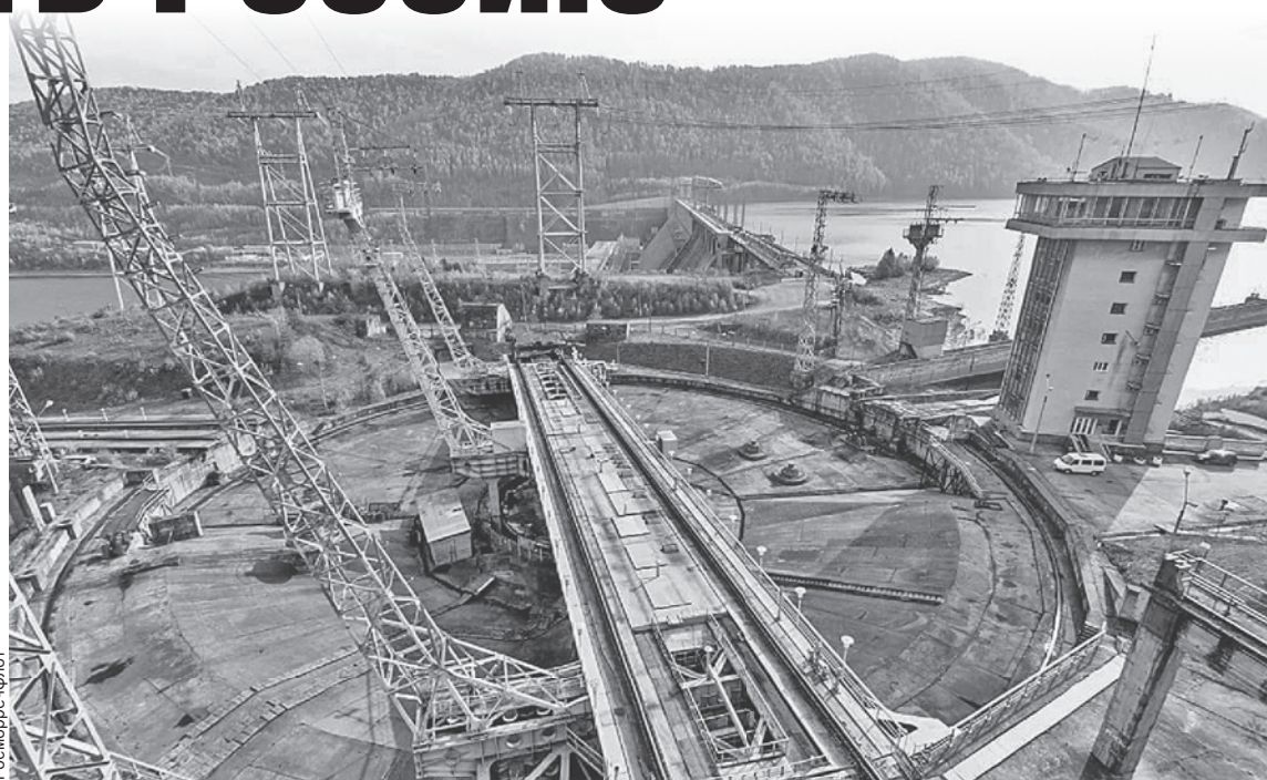
Поворотное устройство Красноярского судоподъемника.
