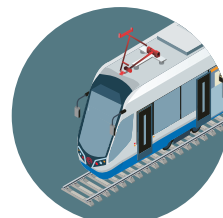
Трамваи
